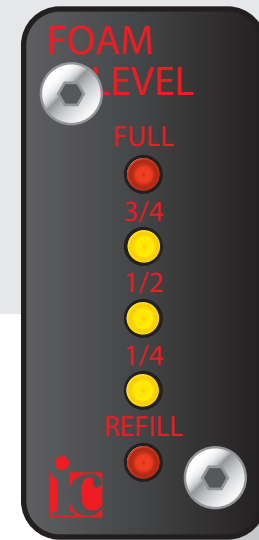
5-LED Mini Slave Foam Display P/N 3030420
