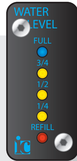
5-LED Mini Slave Water Display P/N 3030418
